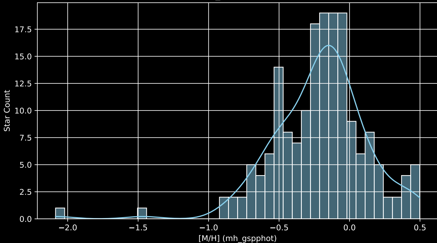
APOGEE DR17 Field: [350+87 MGA [M/H] (mh_gspphot) (n= 178)
